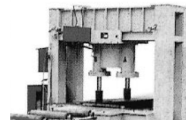
敷鉄板曲がり矯正プレス
